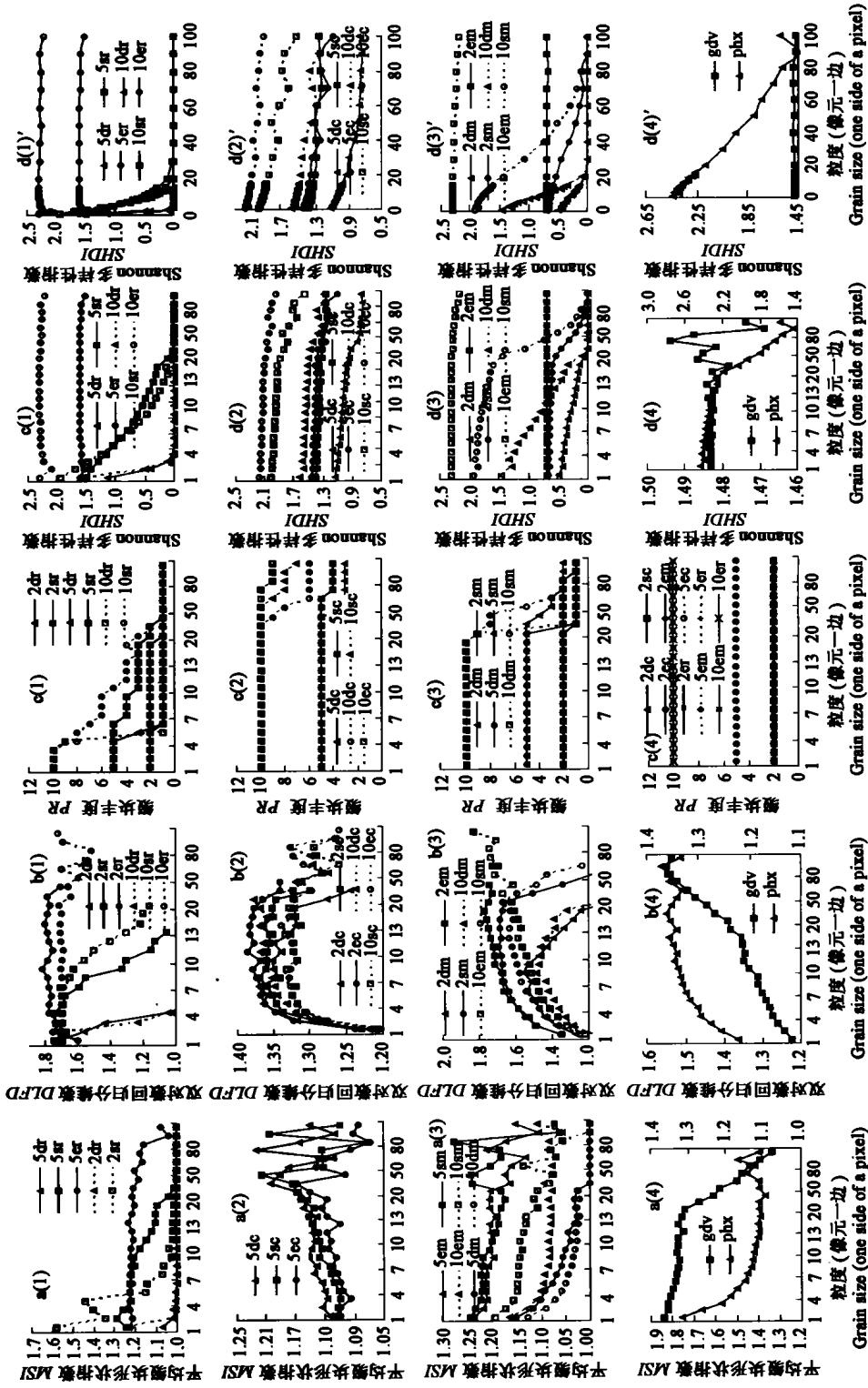
图 4 第 2 类景观指数随空间粒度的变化
