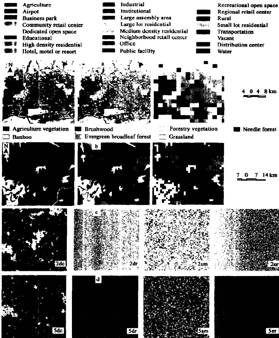
图 1 本研究中所用真实景观与模拟景观举例
